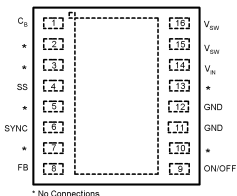
LLP Package
